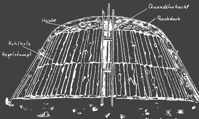
Querschnitt durch den Meiler
